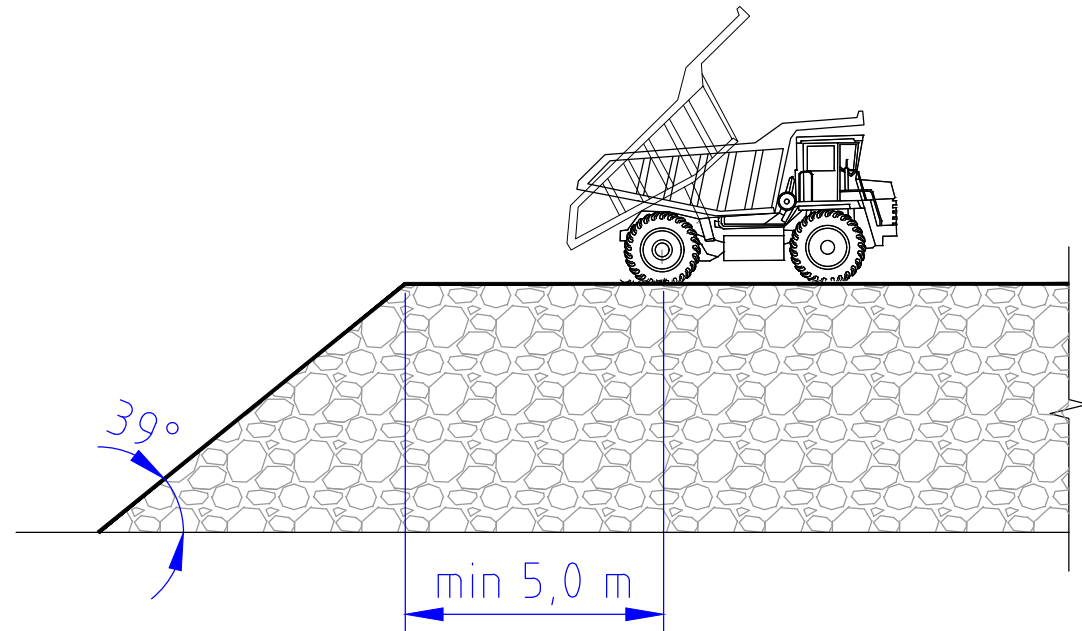
Положение 2. При отсутствии предохранительного вала
