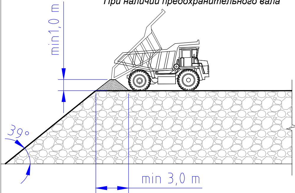
Положение 1. При наличии предохранительного вала
